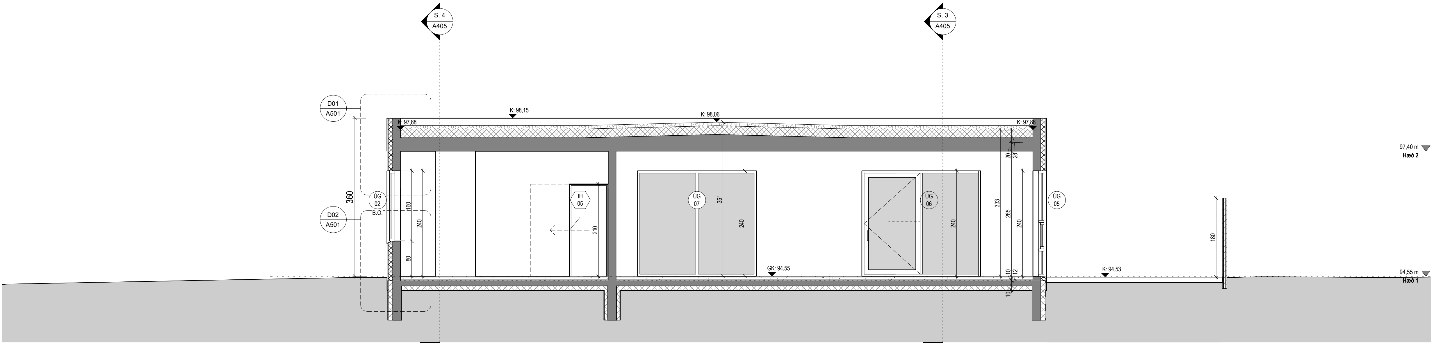
Snið 1 1 : 50
