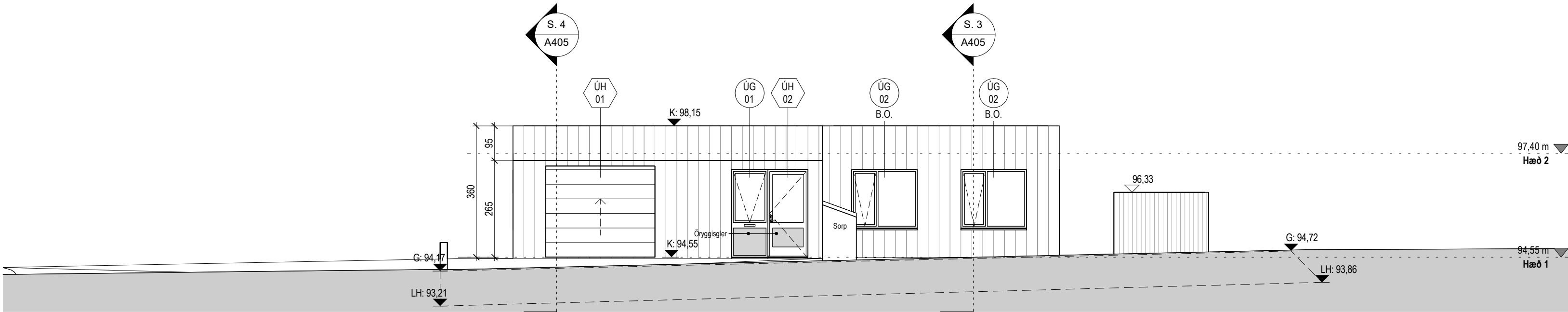
Norðvestur útlit 1 : 100
