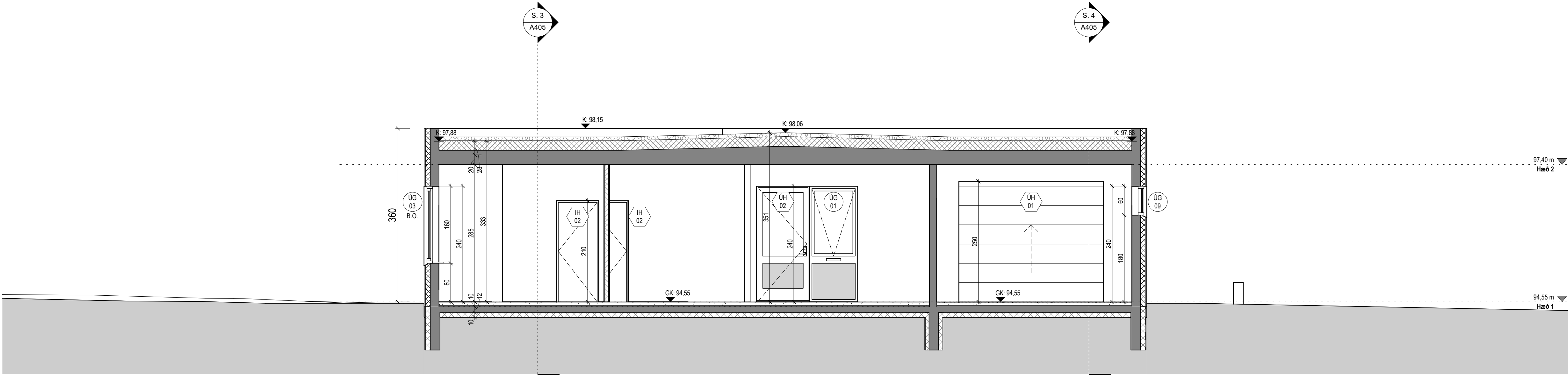
Snið 2 1 : 50
